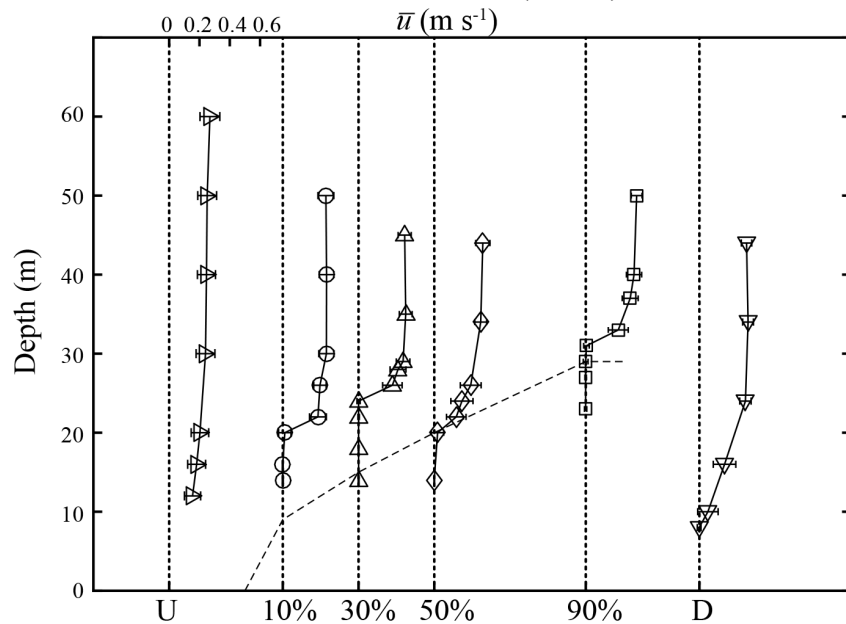
SITE: HV - PATCH N. 6 (L=2.50 m)
